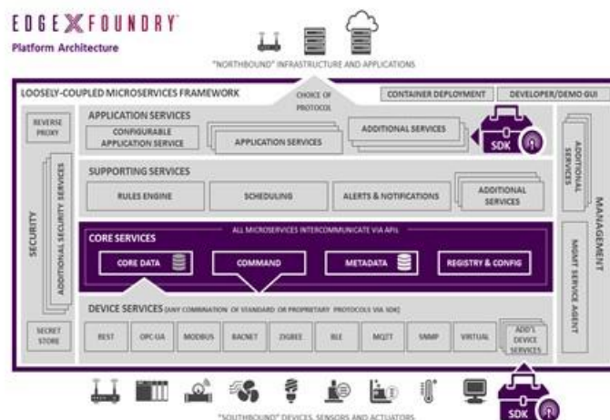
Εικόνα 11: Η Αρχιτεκτονική του EdgeXFoundry
