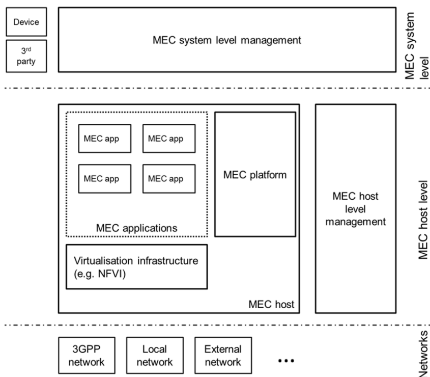
Εικόνα 9: Υψηλού Επιπέδου Αρχιτεκτονική του MEC..
