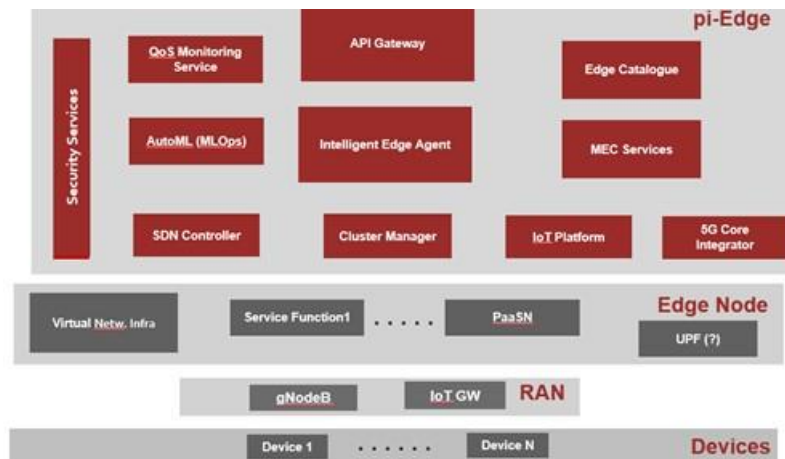
Εικόνα 1: Αρχιτεκτονική υψηλού επιπέδου του Διαχειριστή Πλατφόρμας Άκρων
